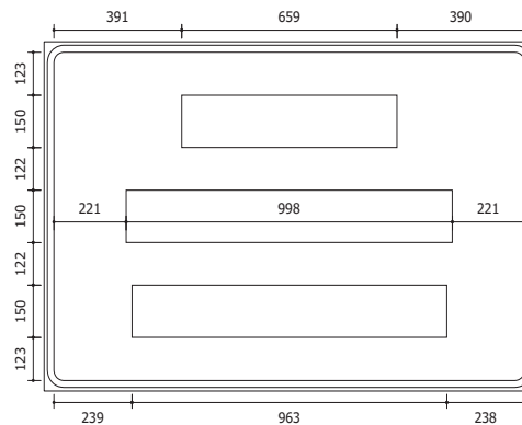
Figura 113 - Desvio à direita a 250 m
