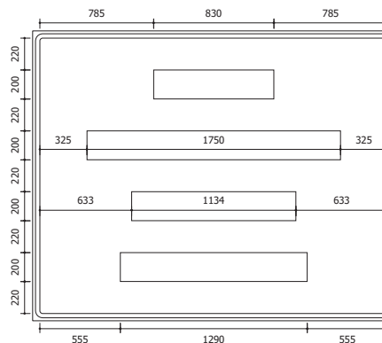
Figura 107 - Obras no canteiro central a 500 m
