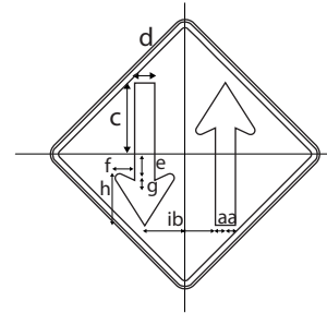
Dimensões (mm)
