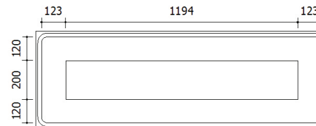
Figura 165 - Placa complementar "A 50 m"
