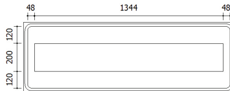
Figura 173 - Placa complementar "A 1,5 km"
