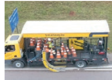
Implantação/Retirada de cones (papa-cones)
