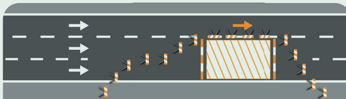
Figura 7 - Esquema de utilização de barreiras Tipo I, II e III
