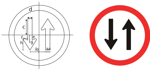
Dimensões (mm)
