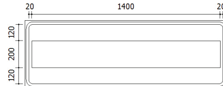
Figura 170 - Placa complementar "A 500 m"
