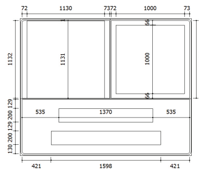
Figura 164 - Placa composta A-24 + R-7 + "Reduza a Velocidade"
