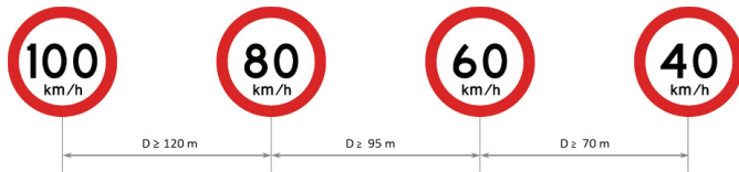
Figura 51 - Distâncias Mínimas necessárias entre placas de velocidade
