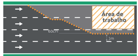
Figura 50 - Posicionamento de dispositivos de canalização – Pista com 4 Faixas (caso 2)
