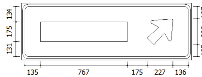
Figura 108 - Desvio à direita
