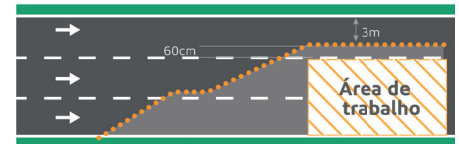
Figura 47 - Posicionamento de dispositivos de canalização – Pista com 3 Faixas (caso 1)
