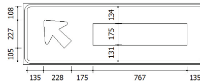
Figura 109 – Desvio à esquerda
