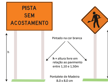
Figura 17 - Placas em pontaletes de madeira
