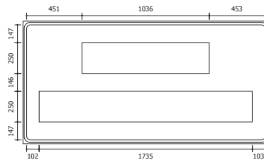
Figura 104 - Obras a 1000 m
