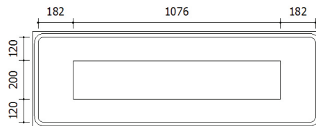
Figura 172 - Placa complementar "A 1 km"
